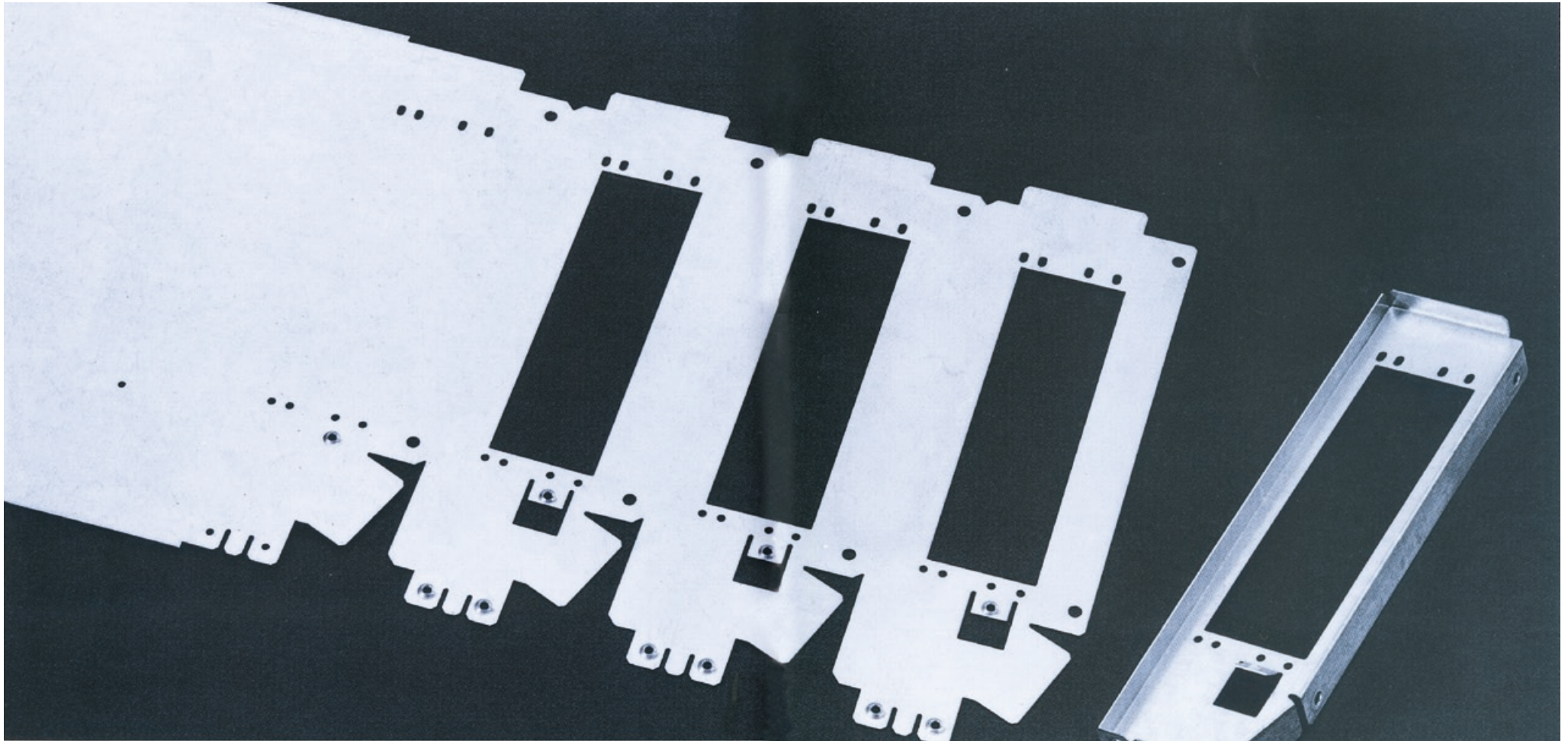
Lüfterträger im Folgebund-Werkzeug gefertigt
