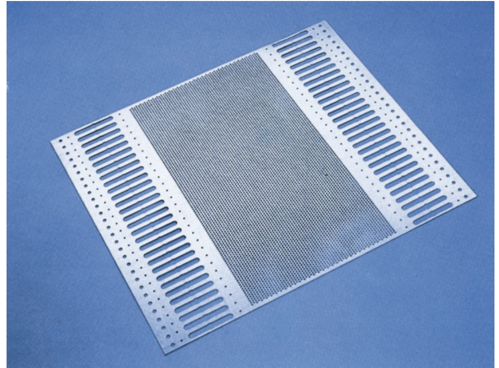
Rückwand für Schaltschrank
